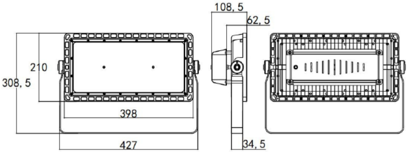
直式支架 單位 mm
